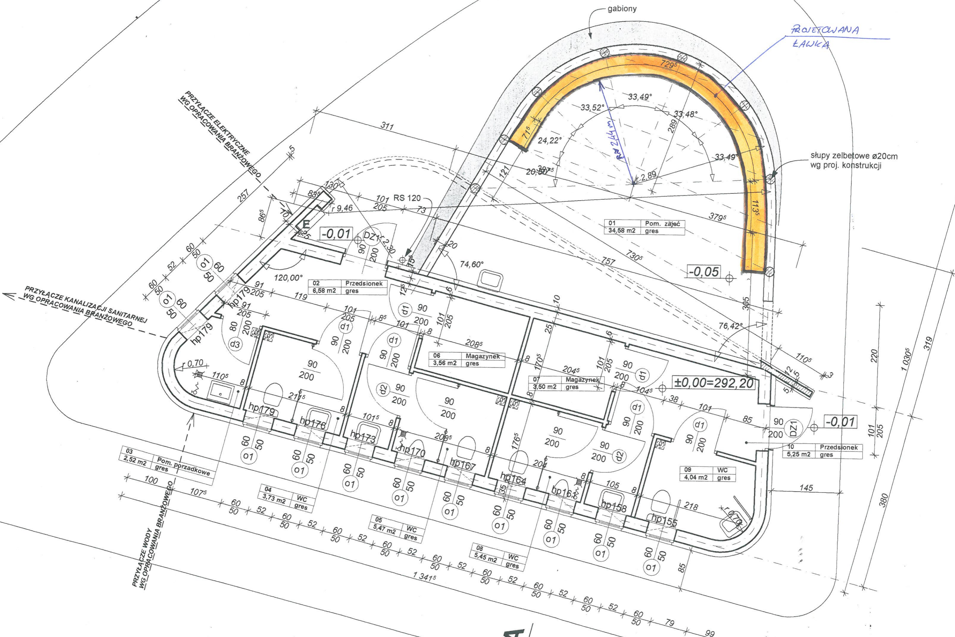
RZUT PARTERU
